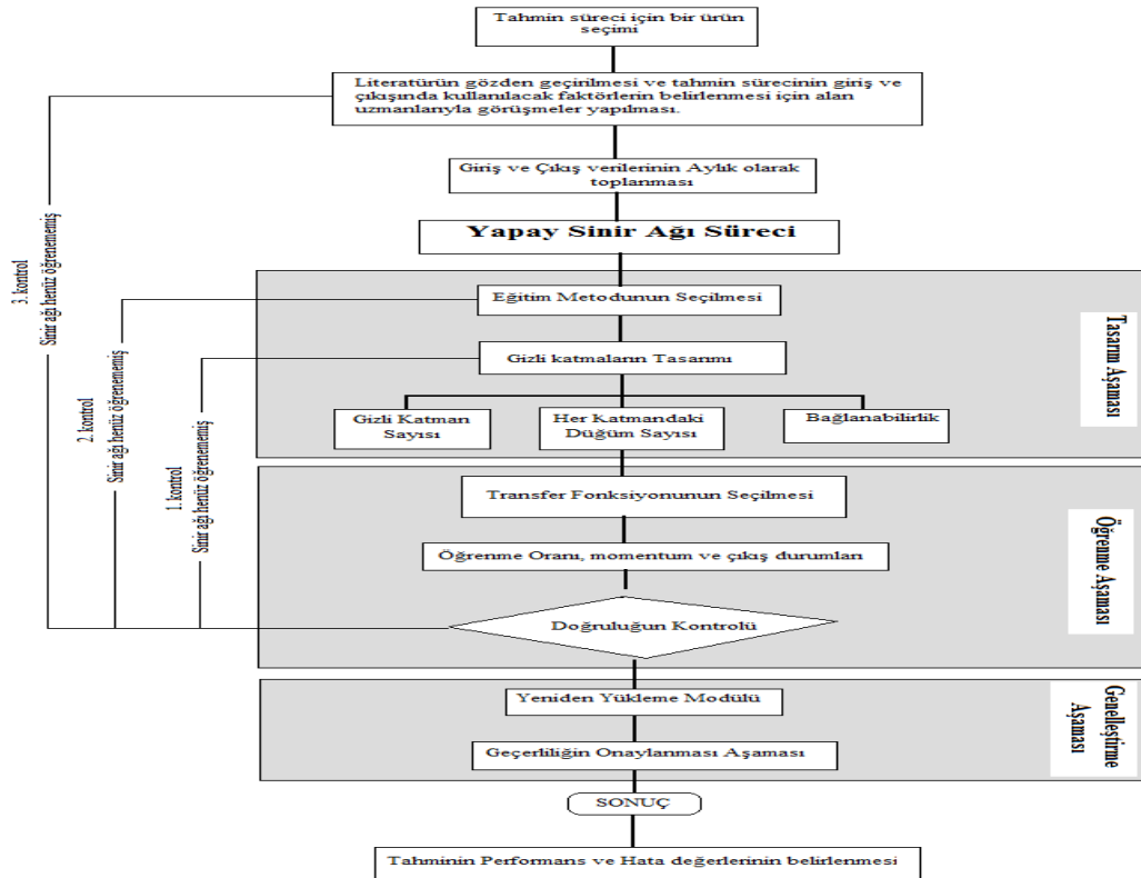
Şekil 2. Yapay Sinir Ağı Modelinin Tasarım Süreci
